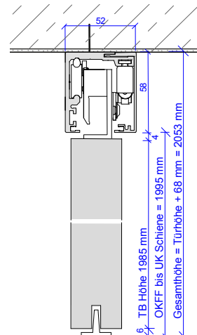
Deckenmontage
