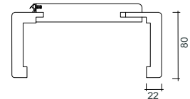
Futter Rundform (RF), Bekleidungsbreite 80 mm
