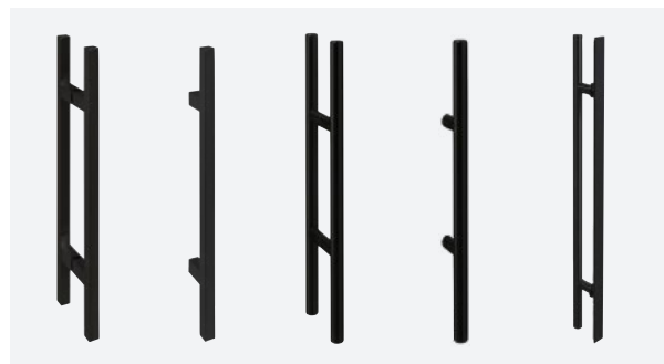
Standard eckig beidseitig Standard eckig einseitig Standard rund beidseitig Standard rund einseitig Standard rund, einseitig Flachstahl Paar / 600 mm Paar / 600, 1200 mm Paar / 400, 600 mm Paar / 400, 600 mm Paar / 400 mm
