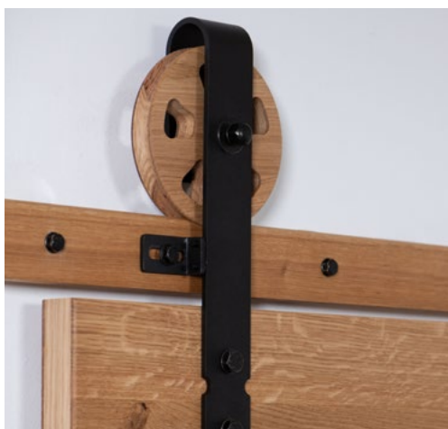
Detail Laufrolle
