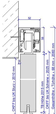
Wandmontage, ohne Futter
