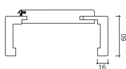
Futter Kleine Rundkante (KR), Bekleidungsbreite 60 mm
