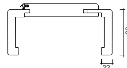
Futter Rundform (RF), Bekleidungsbreite 80 mm
