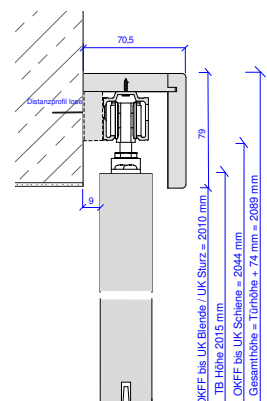
Außenlaufend, ohne Futter
