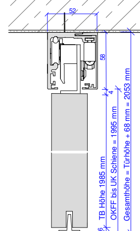
Deckenmontage
