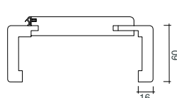
Futter Rundform (RF), Bekleidungsbreite 60 mm
