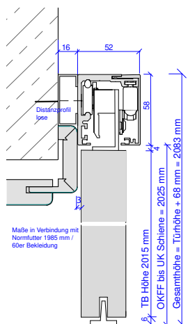
Wandmontage, mit Futter
